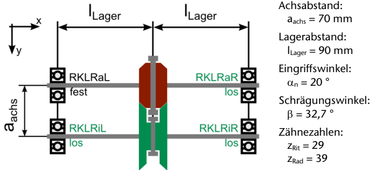
Abbildung 4: Skizze des Beispielgetriebes: Variante 3 mit Rillenkugellagern und Druckkamm Lagerung. Das einzige Festlager dieser Variante dient lediglich als Führungslager, eine axiale Belastung aus der Verzahnung erfolgt nicht.
