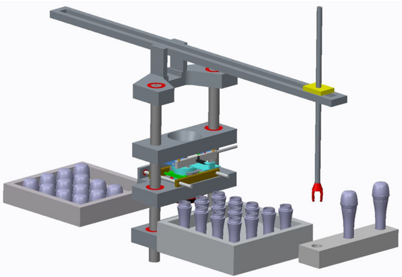
Abbildung 4: Vollständige Fügeanlage
