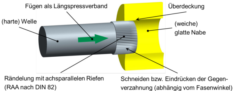
Abbildung 1: Charakteristika einer Pressverbindung mit gerändelter Welle
