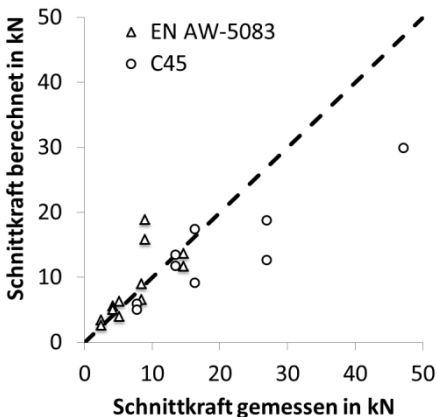
Abbildung 3: Vergleich zwischen berechneter und gemessener Schnittkraft im 45^\circ -Diagramm
